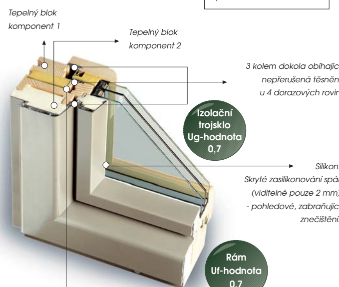
Žádné viditelné izolační vrstvy v oblasti přehybu
