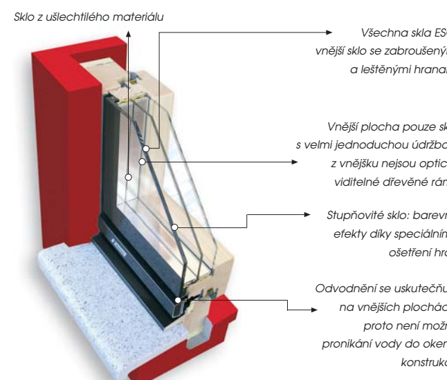
Nosná konstrukce dřevo ve spojení s tepelně izolačními vložkami pro lepší tepelnou izolaci - vhodné také pro pasivní domy
