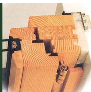
Z vnější strany zakrytý gumou, uvnitř zapěnovaný PU-pénou
