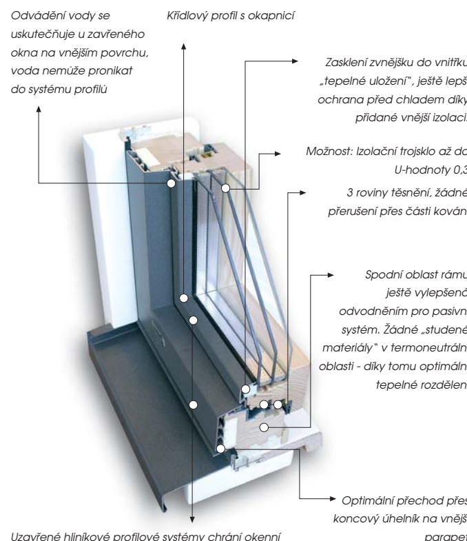
Uzavřené hliníkové profilové systémy chrání okenní rám před nečistotami a hmyzem. Nutné zadní odvětrání je skryto před okem zákazníka.
