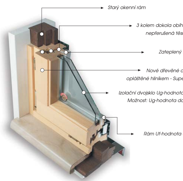
Přírodní materiál dřevo je prodyšné a zaručuje nejvyšší hodnoty tepelné a protihlukové izolace. Díky přidanému opláštění z hliníku mají okna extrémně dlouhou životnost a jsou bezúdržbová. Silber poskytuje 5 let záruku na funkčnost, techniku a těsnost. Díky tomu nabízí Renolux jednoduchou, rychlou a spolehlivou montáž bez dalších vedlejších prací.
