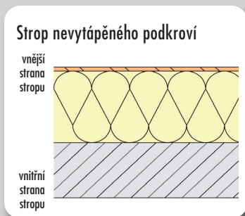
Například – izolace železobetonového stropu
